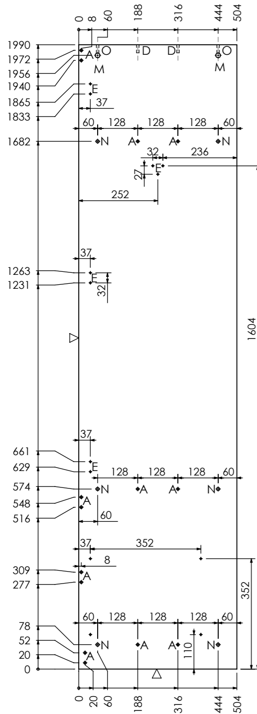
Poz 1 Bočna stranica lijeva
