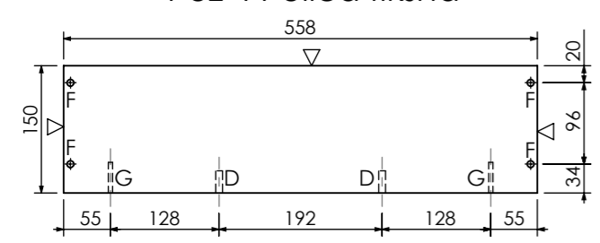
Poz 4 Polica fiksna
