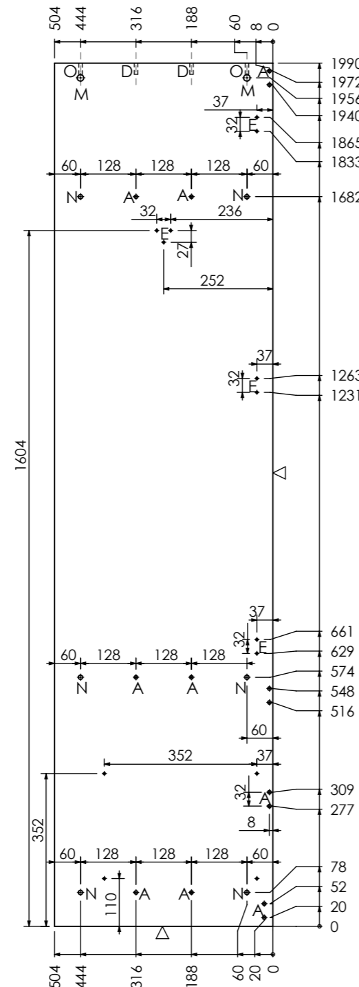
Poz 2 Bočna stranica desna
