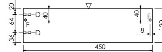
Poz 7 Korpus ladice L/D
