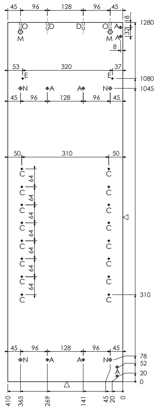
Poz 9 Pomična policica
