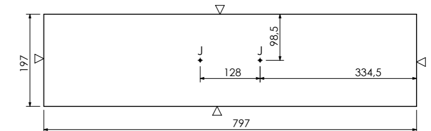
Poz 11 Maska ladice
