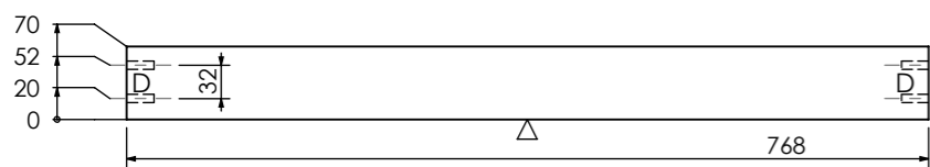
Poz 6 Korpus ladice P/Z
