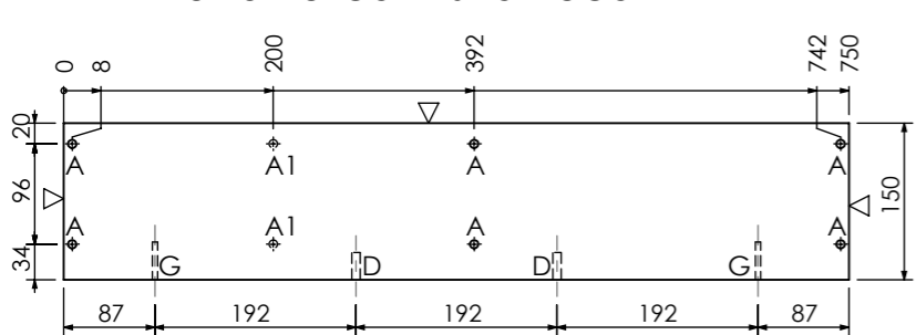
Poz 5 Polica fiksna veca
