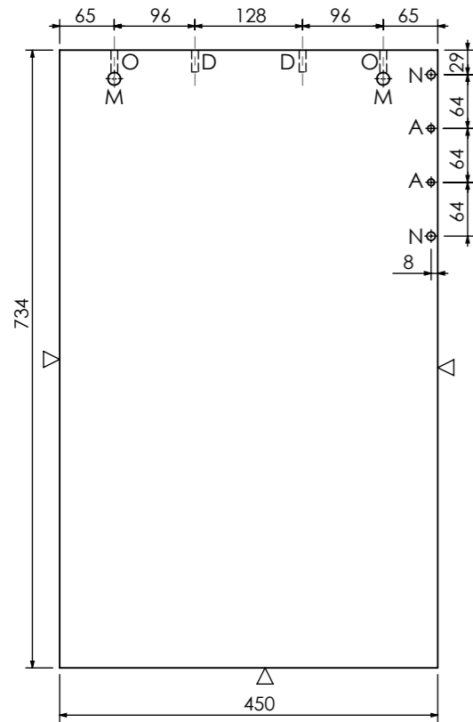
Poz 1 Bočna stranica lijeva
