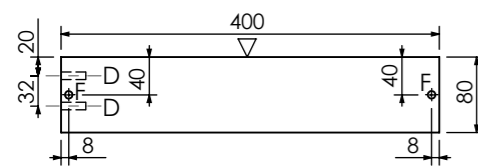
Poz 8 Korpus ladice L/D
