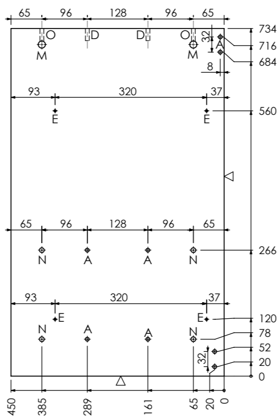
Poz 3 Bočna stranica desna
