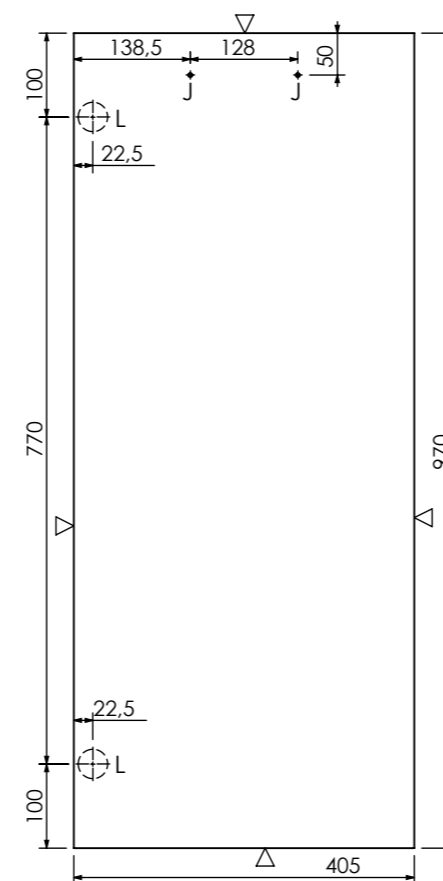
Poz 10 Fronta lijeva
