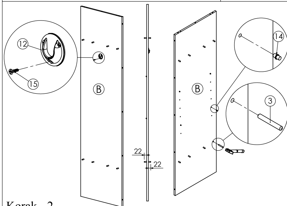
Montaža ORMARA
