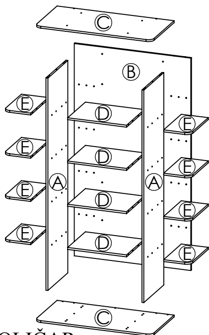
Montaža POLIČAR
