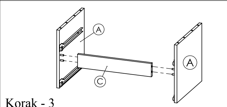
Montaža NOČNIKA
