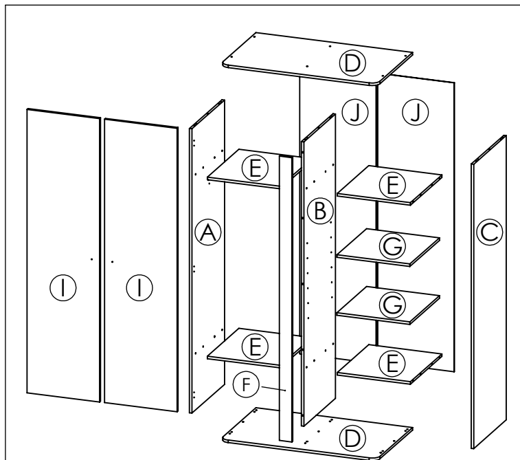
Montaža ORMARA
