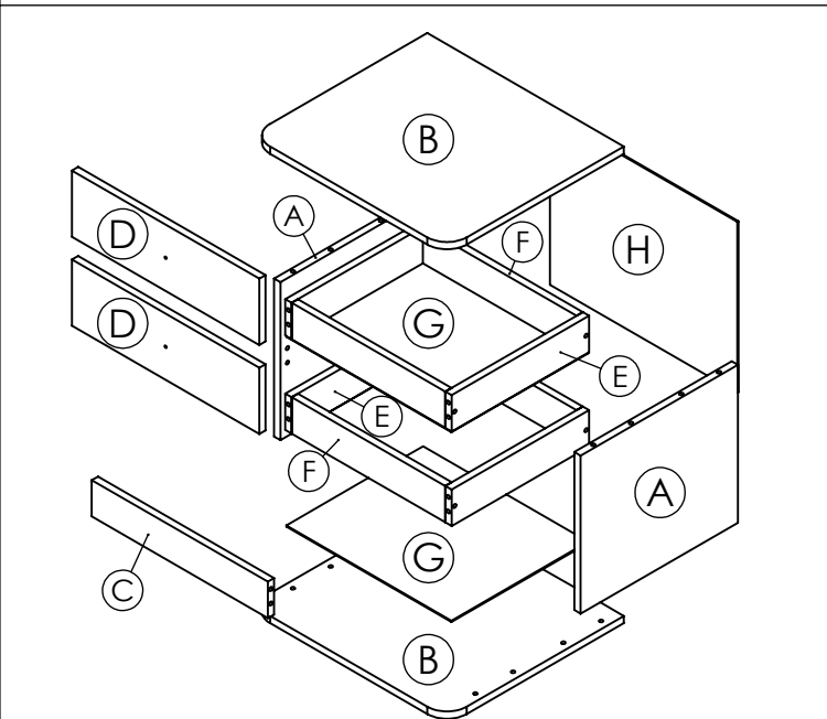
Montaža NOČNIKA
