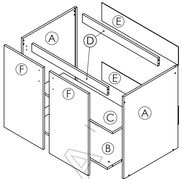
Montaža D-80 Sudoper
