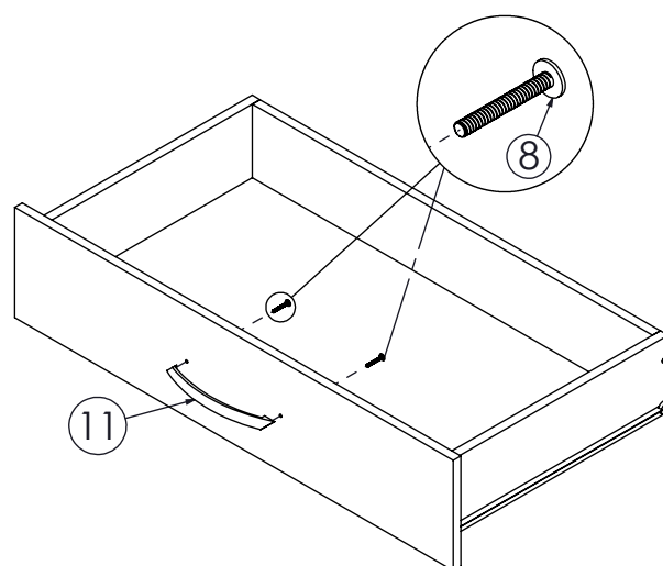
Napomena:lijeva i desna ladica se montiraju na isti način Korak -12-
