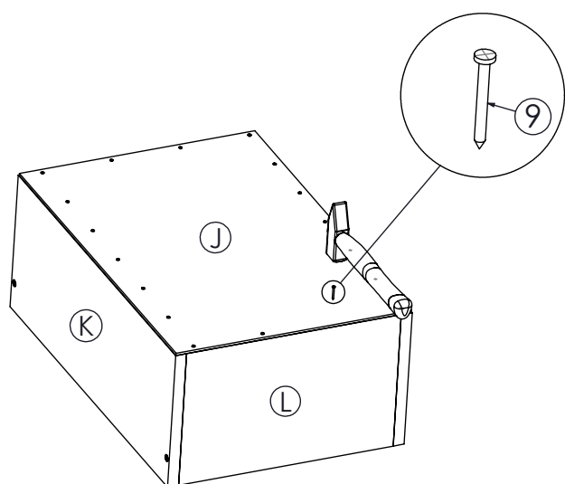
Korak 4
