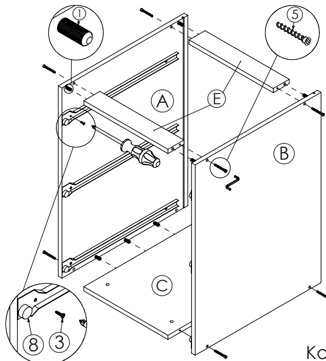
Montaža D-403L
