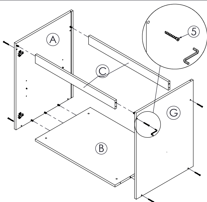
Korak 2
