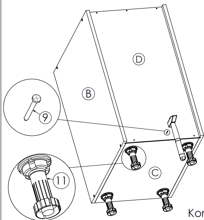
Montaža D-403L
