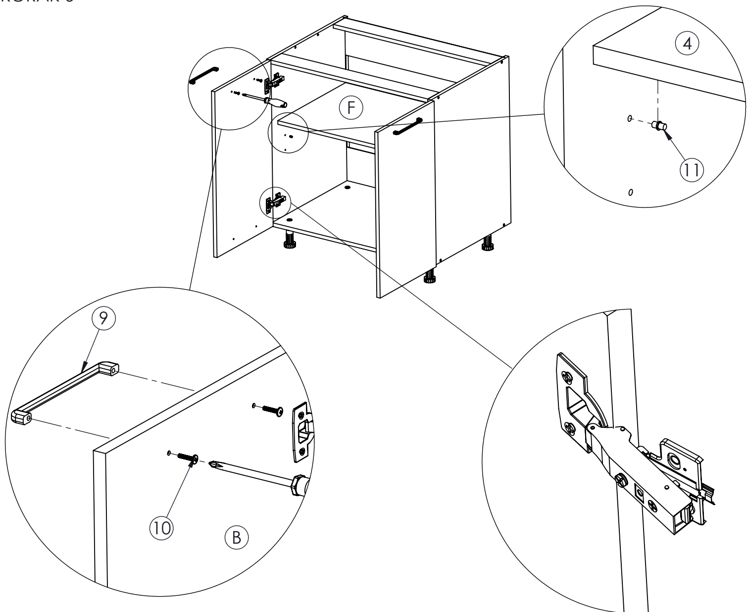
Uklapanje vrata sa podloškom
