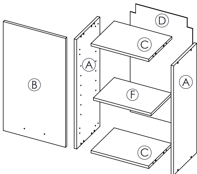
Montaža G-40
